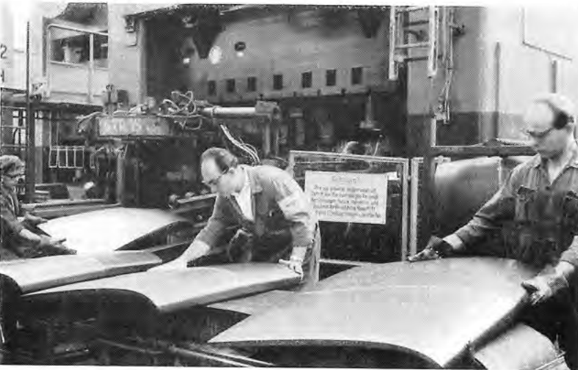
NACHSCHLAGOPERATION bei der Herstellung des Kotflügels auf der Straße 20. (oben)
