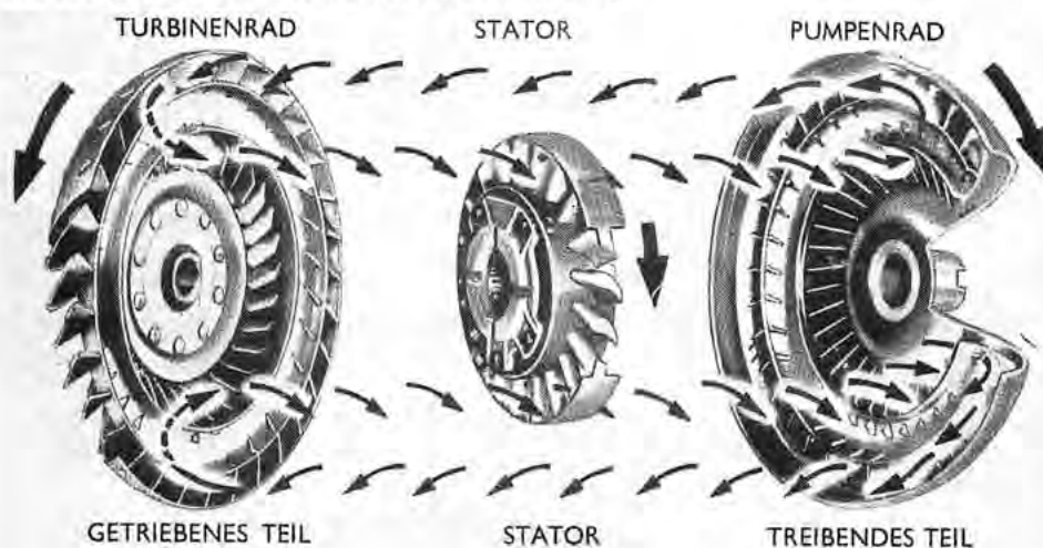
Abb. 2. Der Drehmomentwandler (Stator = Leitrad).
